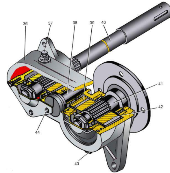
Редуктор цилиндрический подпрессовывающих валльцев
