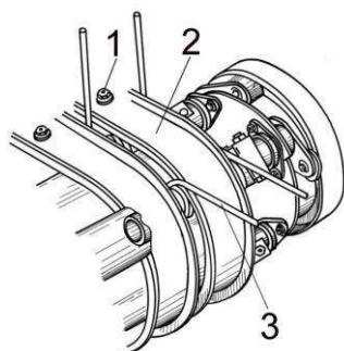
Рисунок 3.21 – Замена пружинного зуба (подборщик ПКК 0350000)
