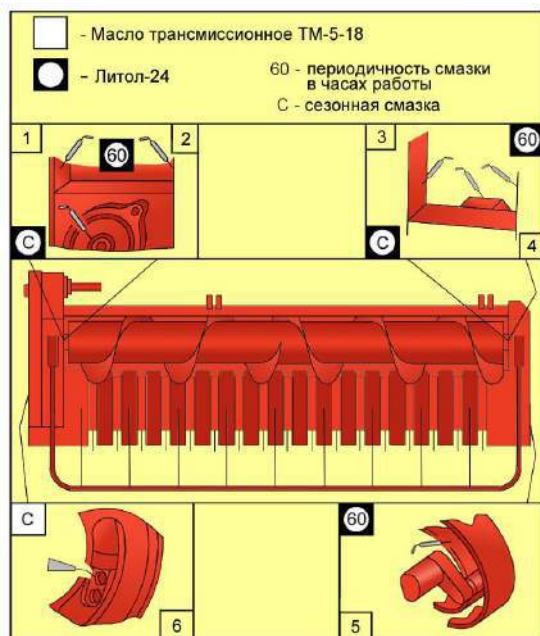
Подборщик ПКК 0350000
