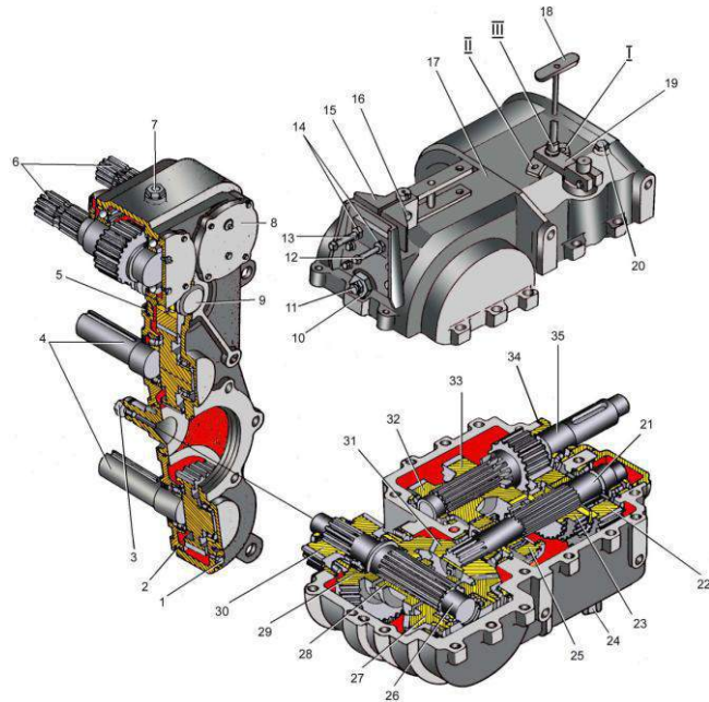
Коробка трехскоростная
