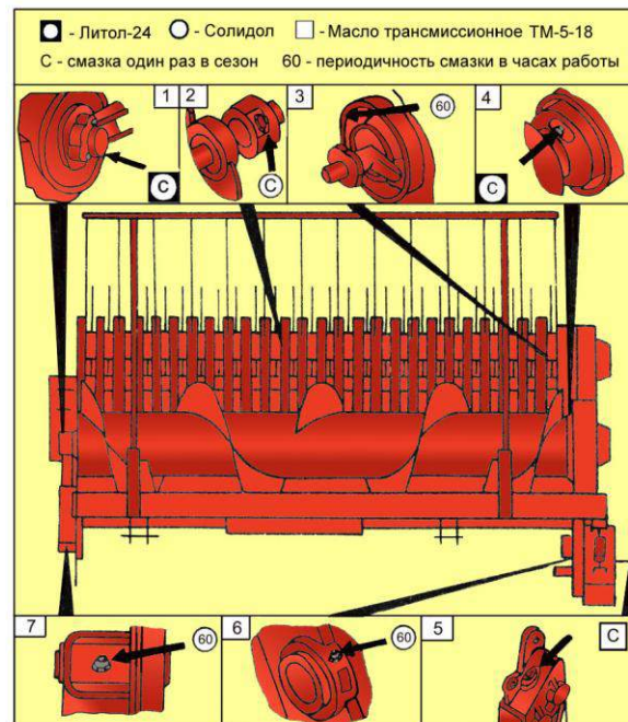
Подборщик ПКК 1900000
