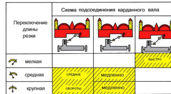
РЕКОМЕНДУЕМЫЕ РЕЖИМЫ РАБОТЫ ЗАШТРИХОВАНЫ
