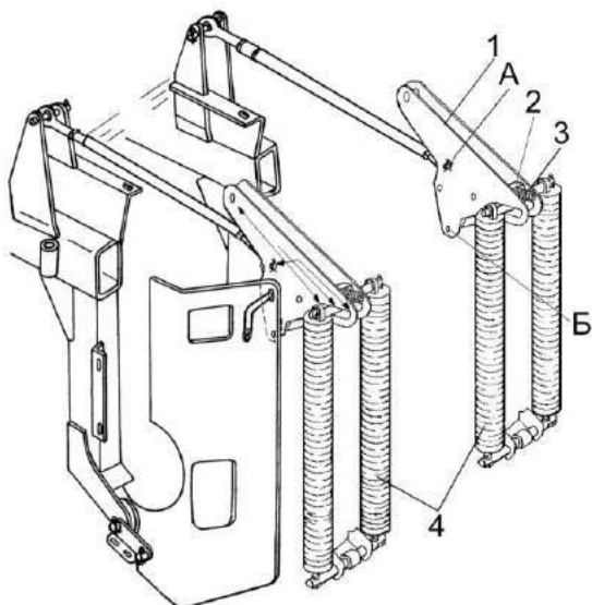
1 – рычаг механизма вывешивания; 2 – серьга; 3 – регулировочный болт; 4 – блок пружин
