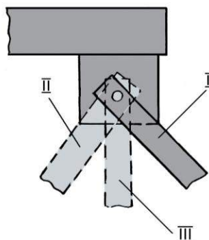
Схема положений сннца относительно рамы комбайна
