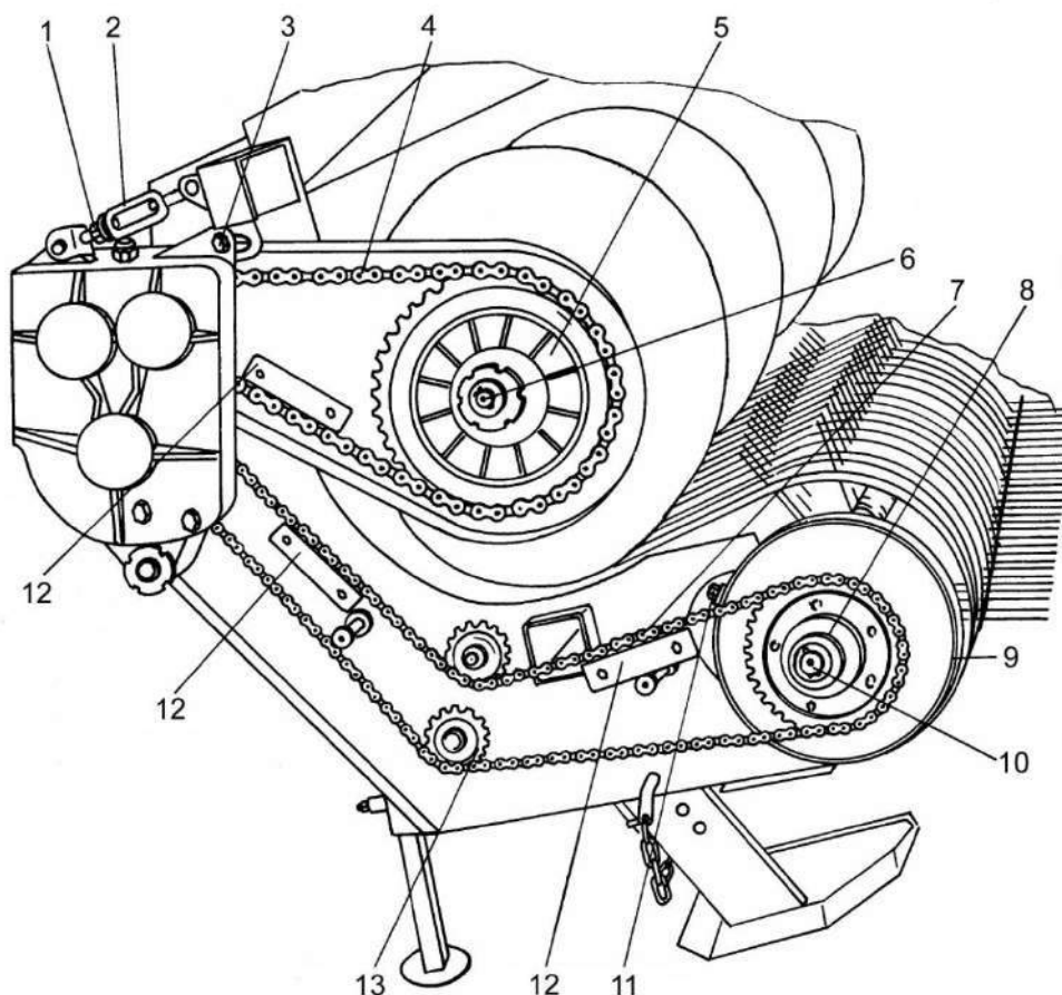
1, 3 – гайки; 2 – стяжка; 4 – цепная передача шнека; 5 – муфта фрикционная; 6 – винт; 7 – цепная передача подбирающего устройства; 8 – муфта обгонная; 9 – дорожка направляющая; 10 – винт; 11 – болт регулировочный; 12 – успокоитель; 13 – звездочка натяжная
