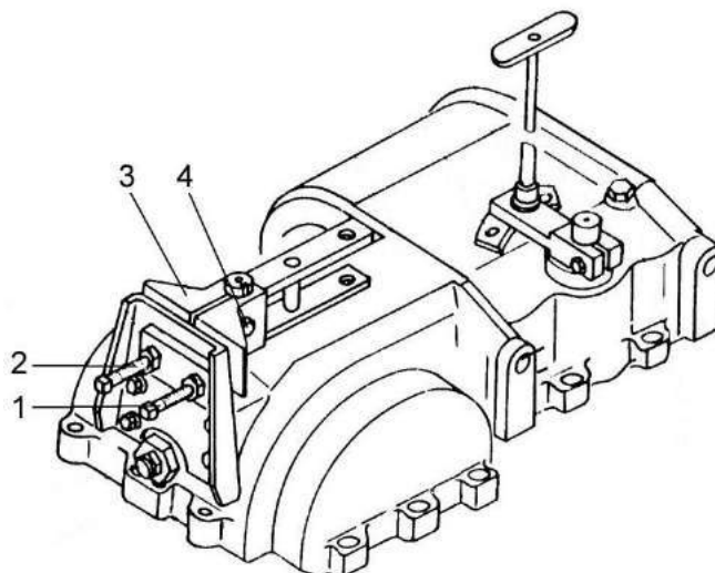
Рисунок 2.4 – Трехскоростная коробка
