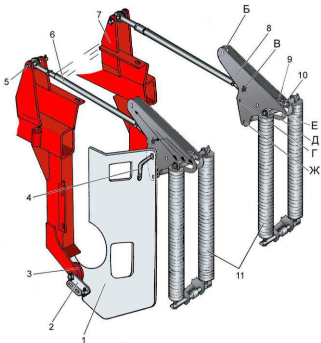
Механизм вывешивания
