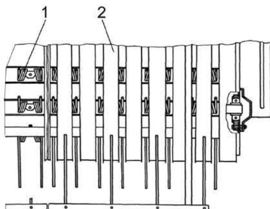
Рисунок 3.20 - Замена пружинного зуба (подборщик ПКК 1900000):
