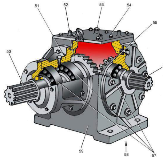
Редуктор конический
