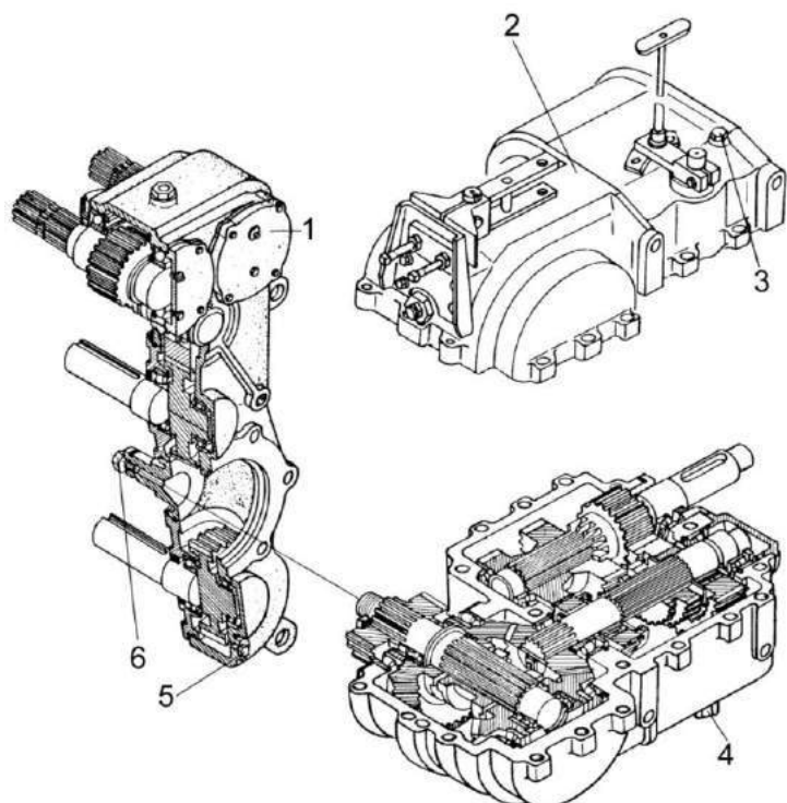
Рисунок 3.9 –Трехскоростная коробка
