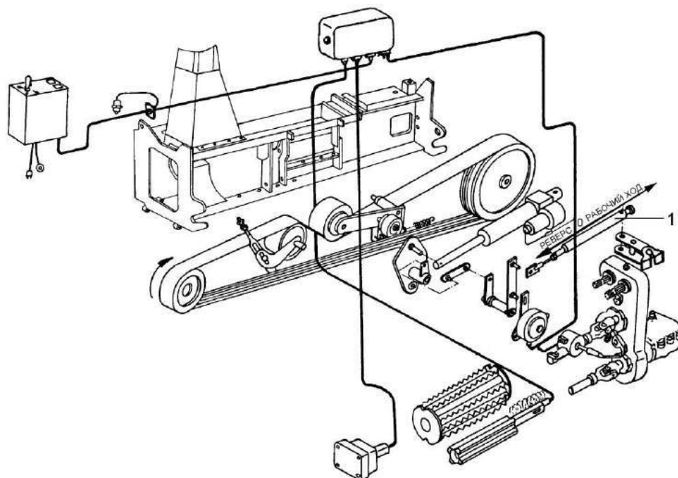
1 – пружинный амортизатор
