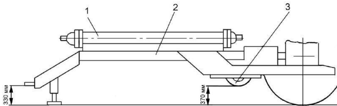
Рисунок 2.11 – Схема подготовки прицепного измельчителя к подсоединению к трактору
