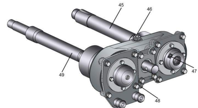
Редуктор цилиндрический подпрессовывающих валльцев
