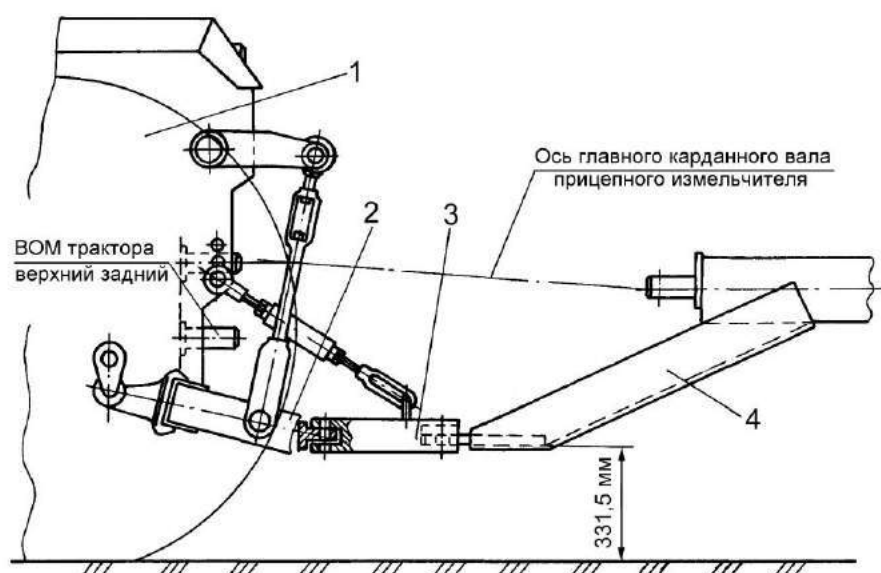
Рисунок Е.1 – Схема подсоединения прицепного измельчителя к трактору ЛТЗ-155
