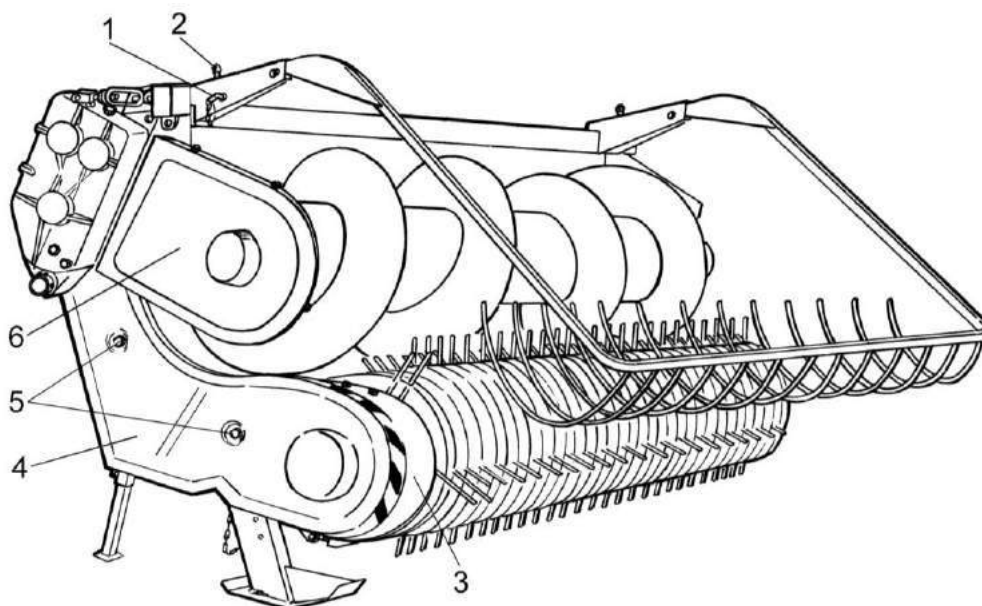
1 – рукоятка; 2 – регулировочный болт; 3 – стяжка; 4 – ограждение; 5 – болты; 6 – крышка рычага
